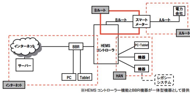
※HEMSコントローラ機能とBBR機器が一体型機器として提供されることもあり得る 12
