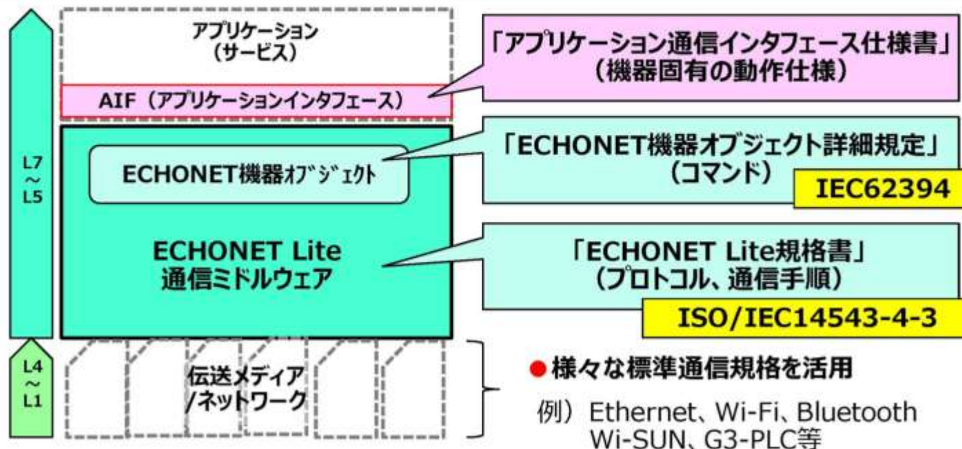
ECHONET Lite プロトコルスタック
